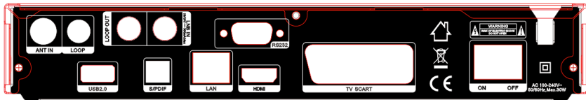
Abbildung 3. Rückplatte
