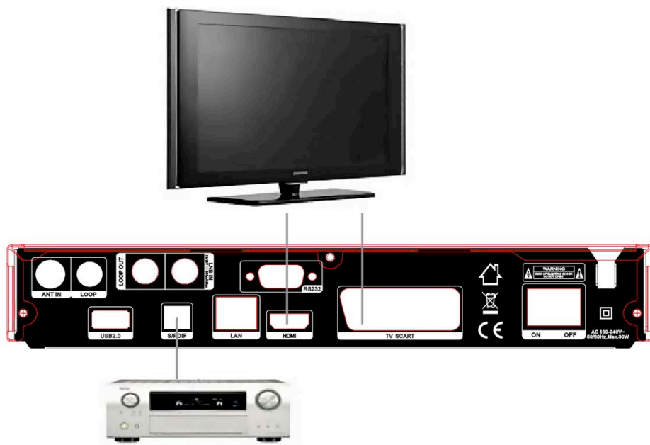
Abbildung 5. Verbindung mit TV & VCR
