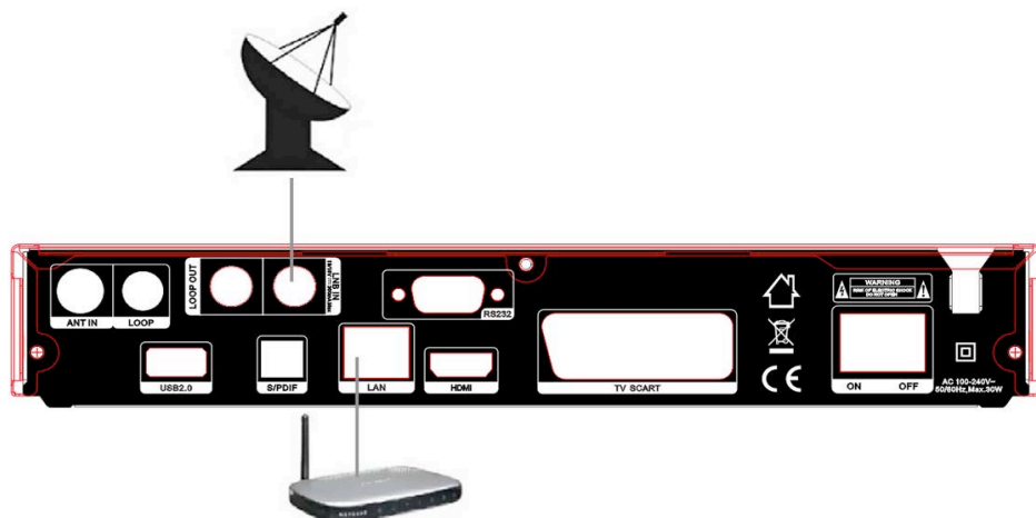
Abbildung 6. Verbindung mit LNB
