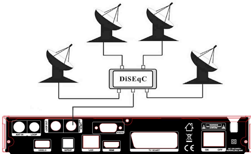
Abbildung 7. Verbindung mit LNB mit Hilfe von DiSEqC
